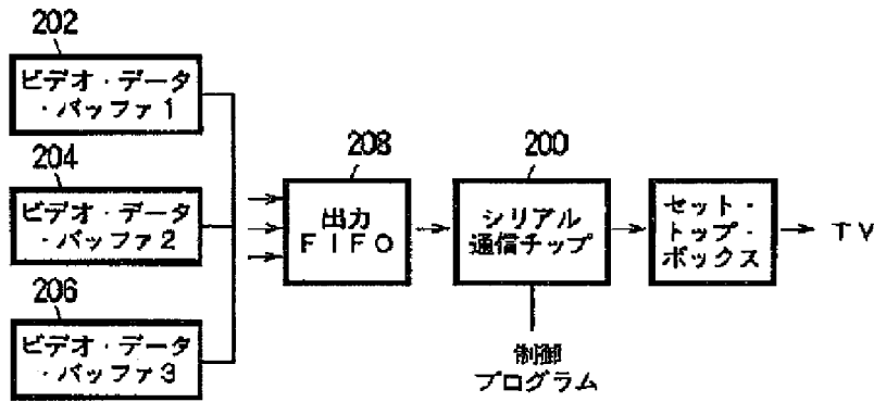
ビデオ通信出力
